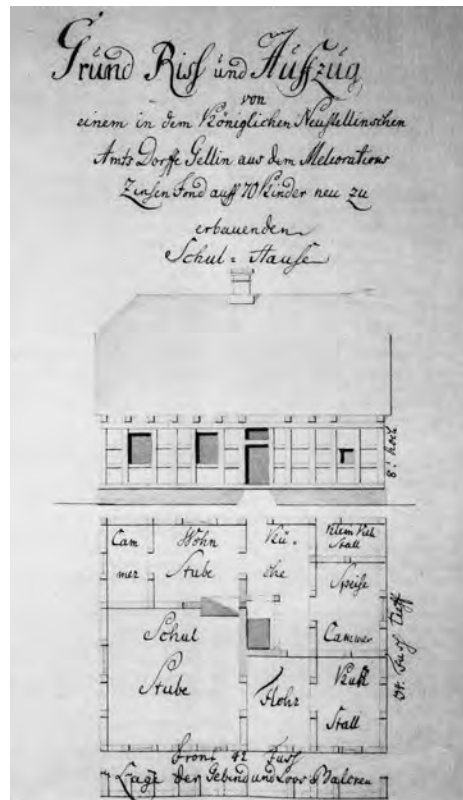
Bild 24: Grundriß von einem im königlichen Amtdorf Gellin zu erbauenden Schulhaus vom 26.02.1780
